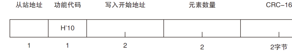
图 13-8 写入多个寄存器 (0x03) 响应帧
