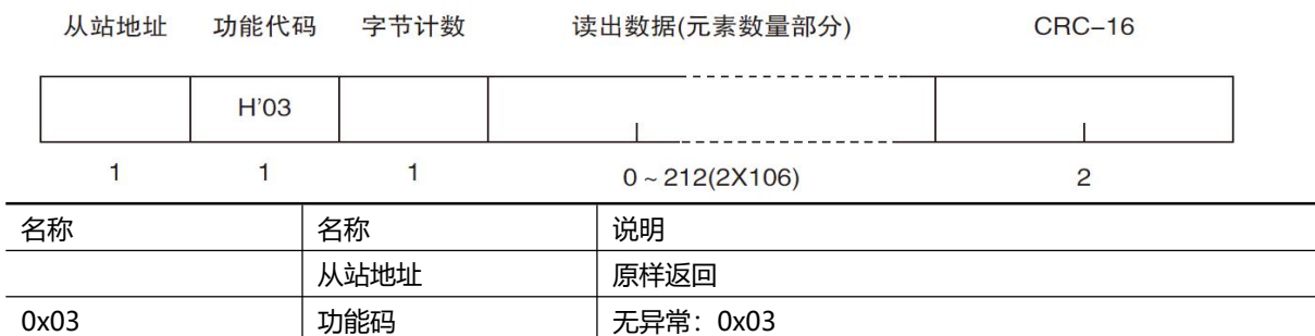
图 9- 5 读出多个寄存器 (0x03) 响应帧
